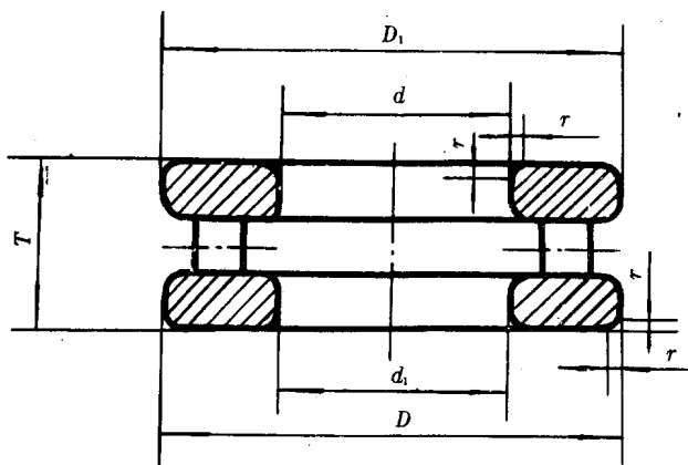
推力圆柱滚子轴承 80000 型
