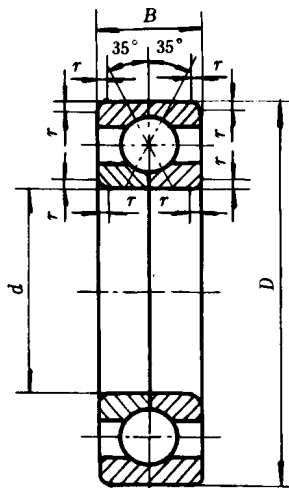
图 2 四点接触球轴承 QJ 型
