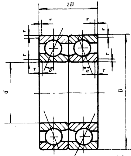
图 8 锁口在内圈上的成对双联 角接触球轴承(面对面) B70000 C/DF 型( \alpha = 15^\circ ) B70000 AC/DF 型( \alpha = 25^\circ ) B70000 B/DF 型( \alpha = 40^\circ )
