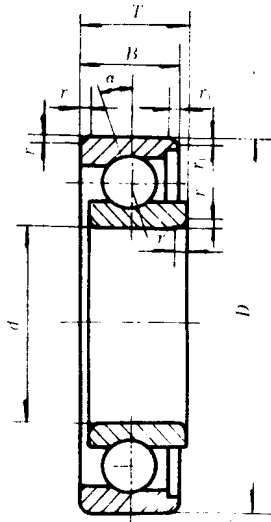
图 1 分离型角接触球轴承 S70000 型( \alpha = 15^\circ )
