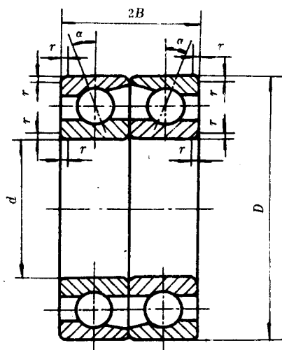
图4 成对双联角接触球轴承 (面对面) 70000 C/DF 型 ( \alpha = 15^\circ ) 70000 AC/DF 型 ( \alpha = 25^\circ ) 70000 B/DF 型 ( \alpha = 40^\circ )
