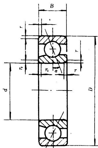
图6 锁口在内圈上的角接触 球轴承 B70000 C 型 ( \alpha = 15^\circ ) B70000 AC 型 ( \alpha = 25^\circ )
