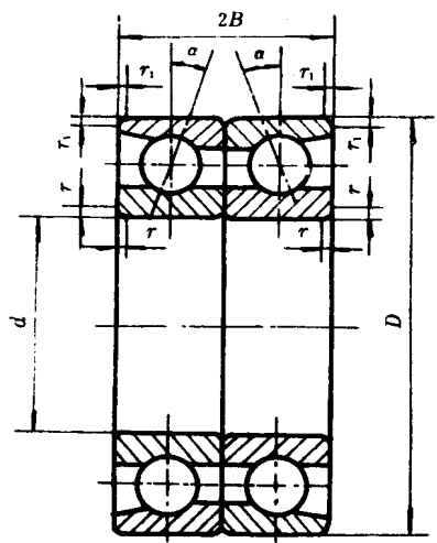
图3 成对双联角接触球轴承 (背靠背) 70000 C/DB 型 ( \alpha = 15^\circ ) 70000 AC/DB 型 ( \alpha = 25^\circ ) 70000 B/DB 型 ( \alpha = 40^\circ )
