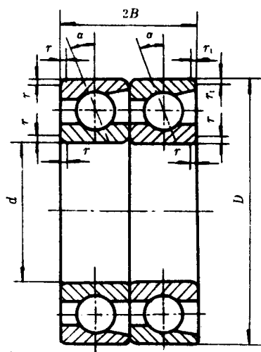
图5 成对双联角接触球轴承 (串联) 70000 C/DT 型 ( \alpha = 15^\circ ) 70000 AC/DT 型 ( \alpha = 25^\circ ) 70000 B/DT 型 ( \alpha = 40^\circ )
