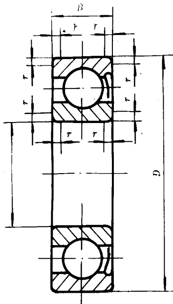
图 4 一面带防尘盖的 深沟球轴承 60000-Z 型
