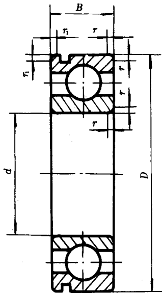
图 2 外圈有止动槽的 深沟球轴承 60000 N 型
