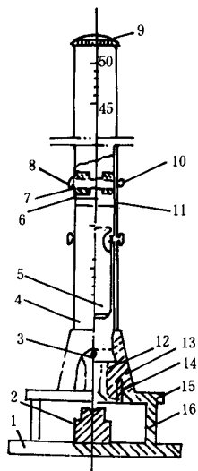
冲击试验器
